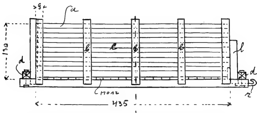
Рис. 7. Боковой видъ баллона (с—боковая стѣнка, п—крюкъ).
